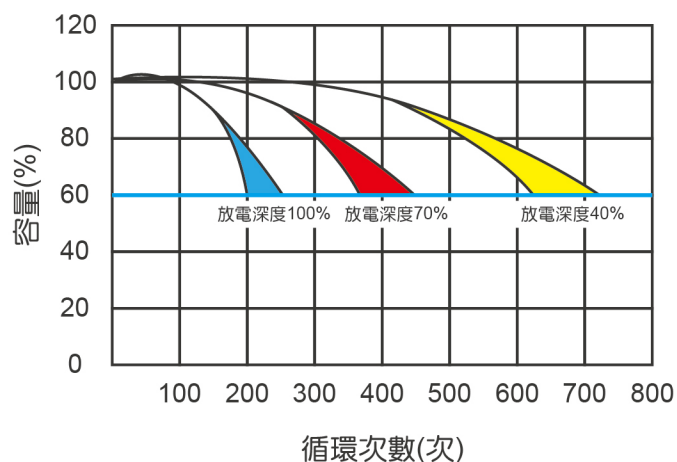
循環使用壽命 (@25°C/77°F)
