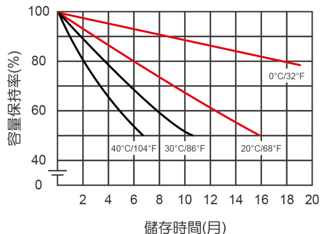
容量保持特性
